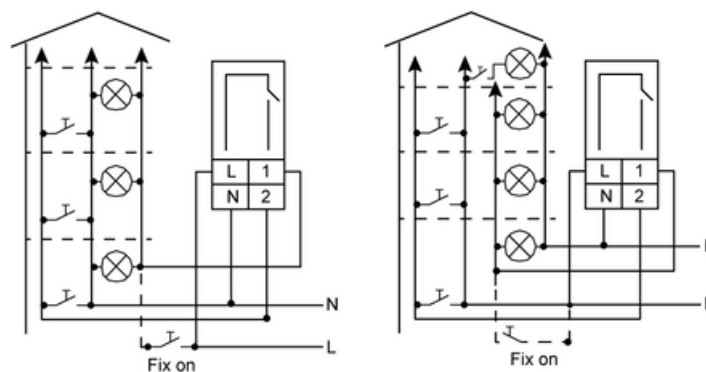
Conexión a 3 hilos 3 wire connection
