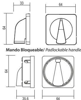
Mando exterior directo Direct external handle
