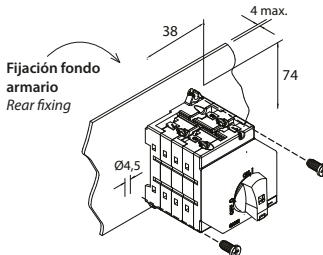
Mando exterior directo Direct external handle
