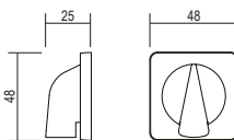
Mando exterior directo Direct external handle
